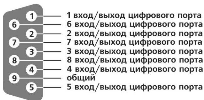
Рисунок А.1 - назначение выводов разъема DB-9 (варианты исполнения ZET 048-С и ZET 048-І)
