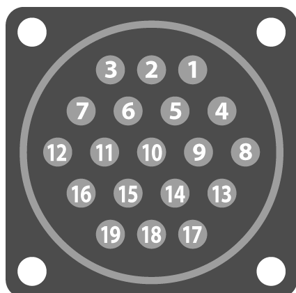
Рисунок А.3 - назначение выводов разъема 2PM24B19Ш1В1 (2PMГ24B19Ш1Е2) (вариант исполнения ZET 048-Е)
