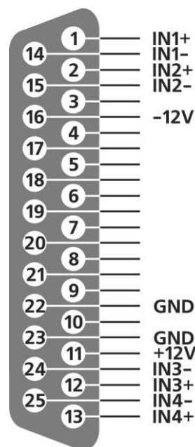
Рисунок А.2 - назначение выводов разъема DB-25 (варианты исполнения ZET 048-С и ZET 048-І)
