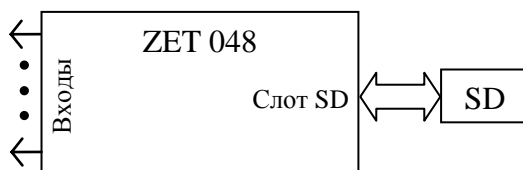
Рисунок 1.10 – подключение регистратора ZET 048-Е при работе в автономном режиме
