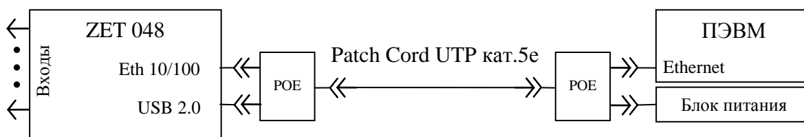
Рисунок 1.6 – подключение регистратора ZET 048-С и ZET 048-И к ПЭВМ по интерфейсу Ethernet с питанием от внешнего источника
