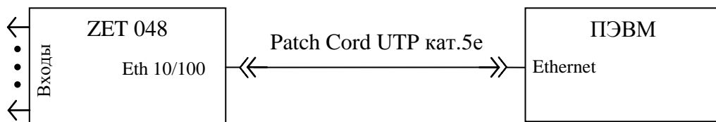
Рисунок 1.8 – подключение регистратора ZET 048-Е к ПЭВМ по интерфейсу Ethernet
