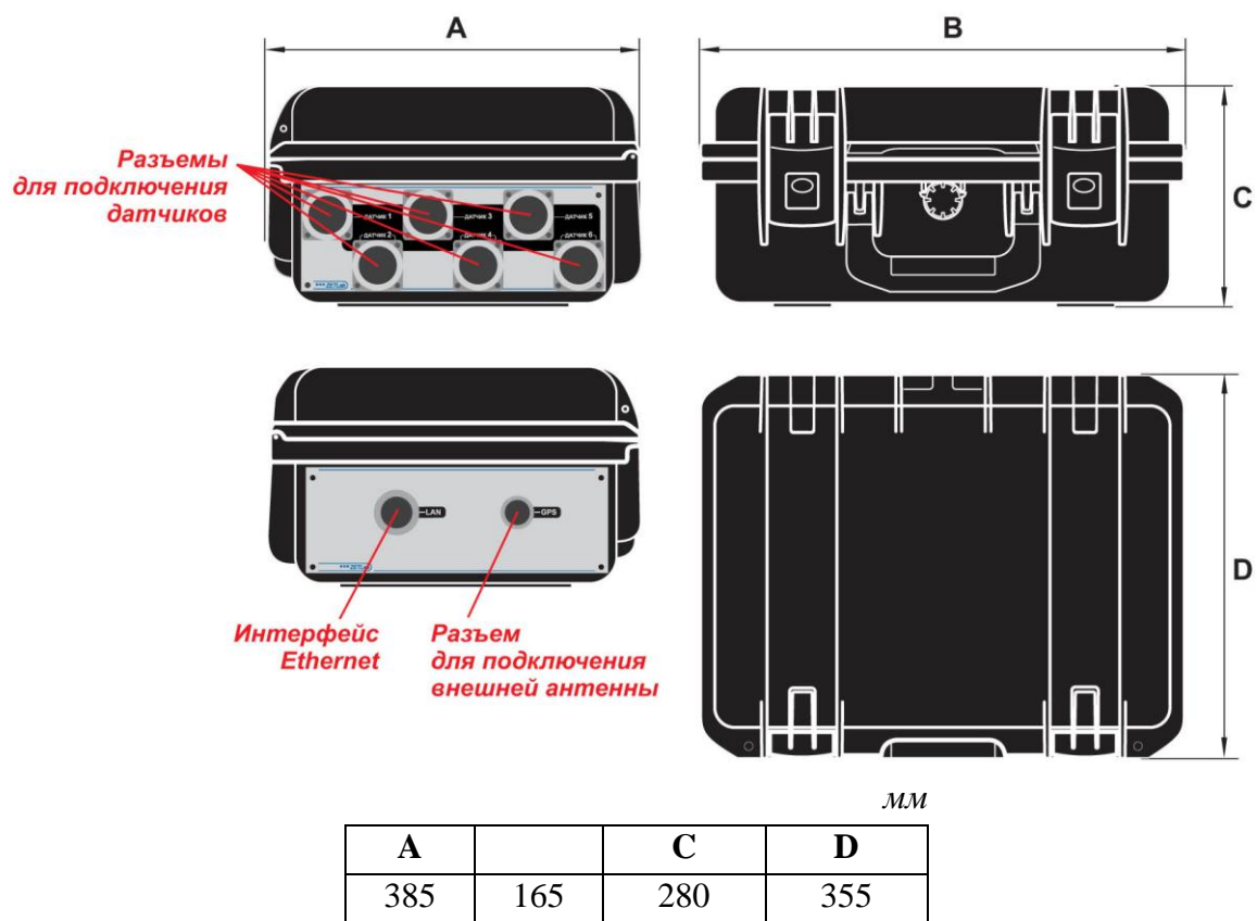
Рисунок 1.3 – общий вид и габариты регистратора ZET 048-E
