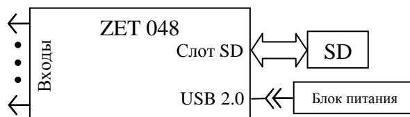
Рисунок 1.9 – подключение регистратора ZET 048-С и ZET 048-И при работе в автономном режиме
