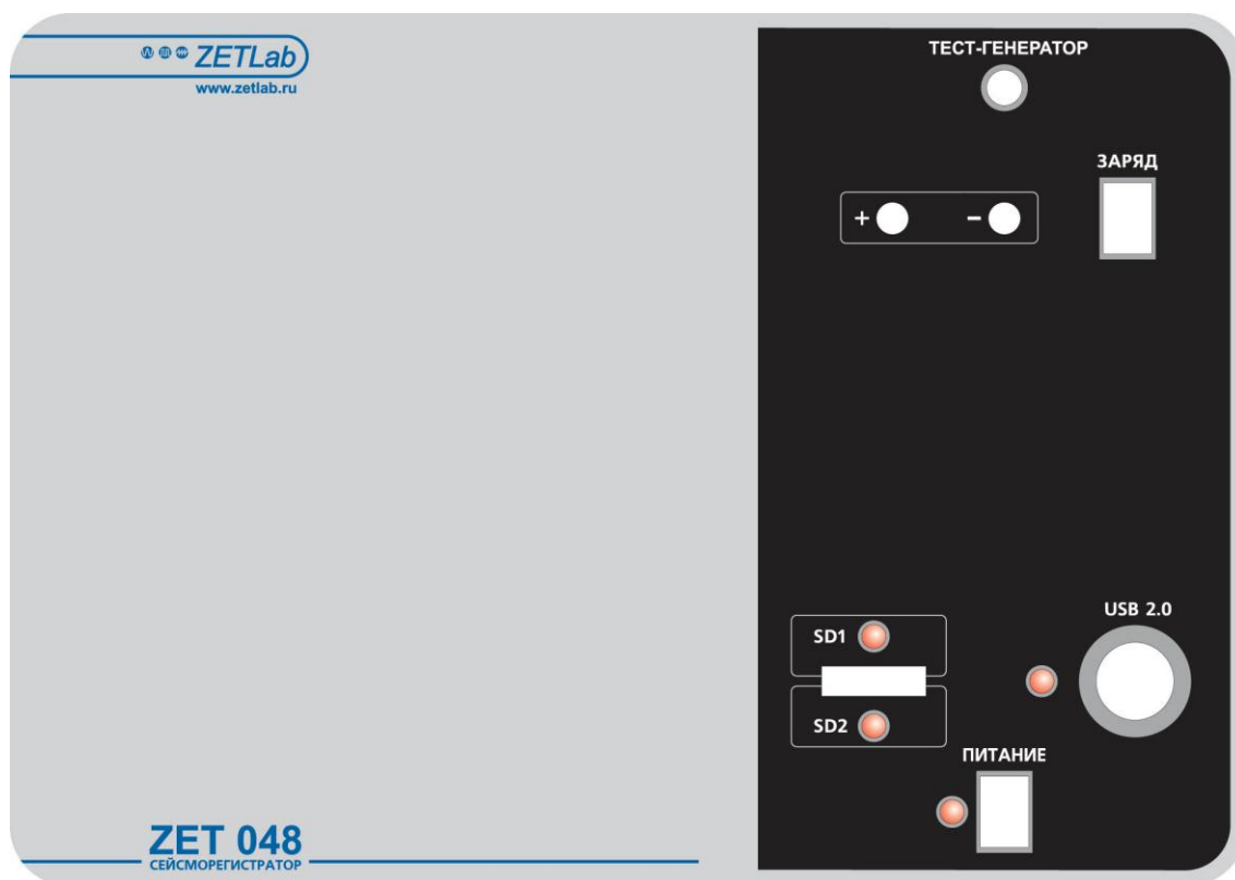
Рисунок 1.4 – панель управления регистратора ZET 048-E
