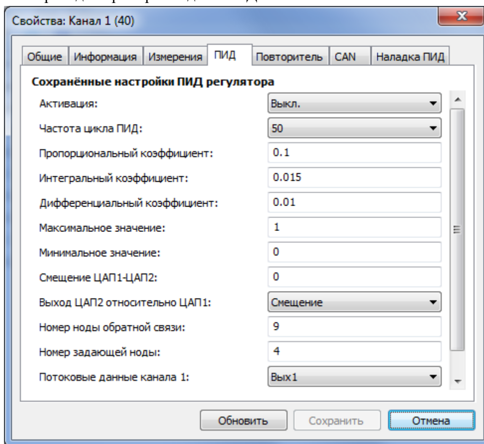
Рис. 4.2 Вкладка «ПИД»
