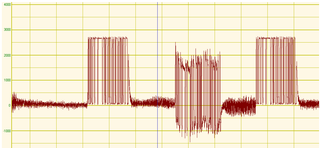
Рисунок 27 Асимметрия сигнала
