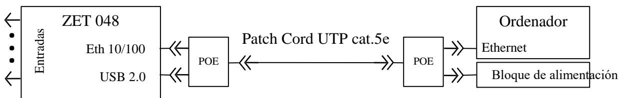
Imagen 1.6 – Conexión del registrador ZET 048-I al ordenador a través de interfaz Ethernet alimentada a través de Ethernet
