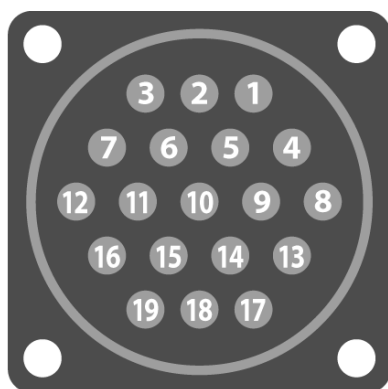
Рисунок А.3 - Назначение выводов разъема 2PM24B19Ш1B1 (2PMГ24B19Ш1Е2) (ZET 048-E)
