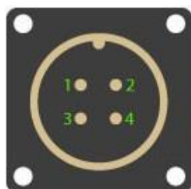
Рисунок А.4 - Назначение выводов разъема FQ14-4ZK (ZET 048-E)
